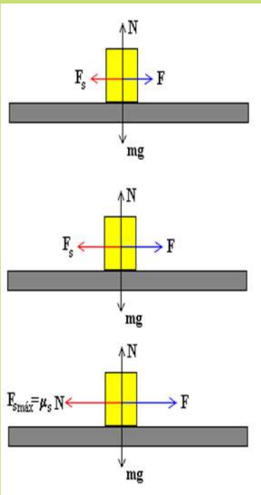
Fuerza de rozamiento cuando el bloque está en reposo
