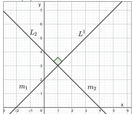
Figura 37: Rectas perpendiculares
