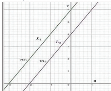
Figura 18 Rectas paralelas
