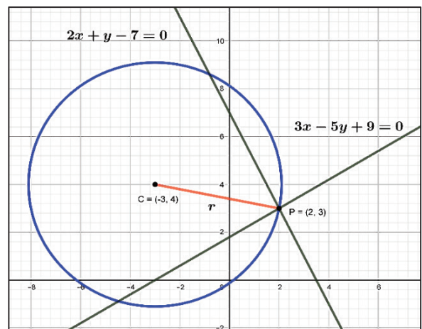
Figura 59 Intersección
