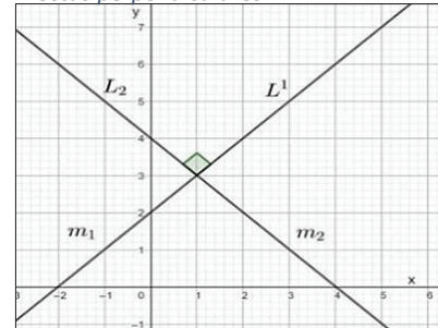
Figura 18 Rectas perpendiculares
