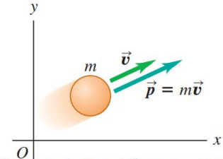
El momento lineal \vec{p} es una cantidad vectorial; el momento lineal de una partícula tiene el mismo sentido que su velocidad \vec{v} .
