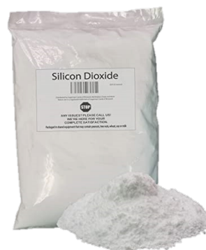
Imagen 6. Anhídrido silíceo
