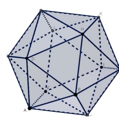
Icosaedro
