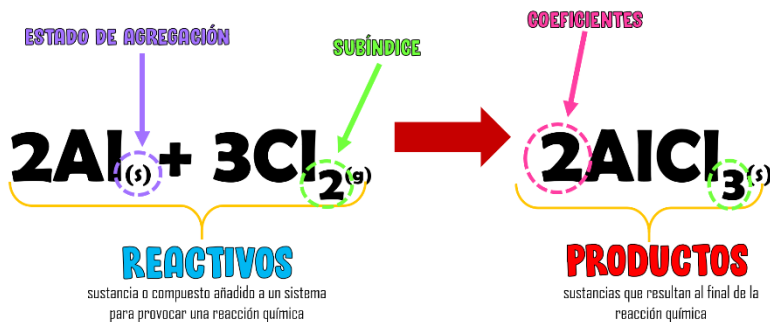
Imagen 2. Reactivos y productos de una fórmula química
