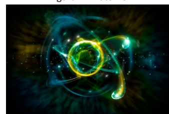
Figura 1: El átomo.
