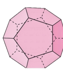
Dodecaedro
